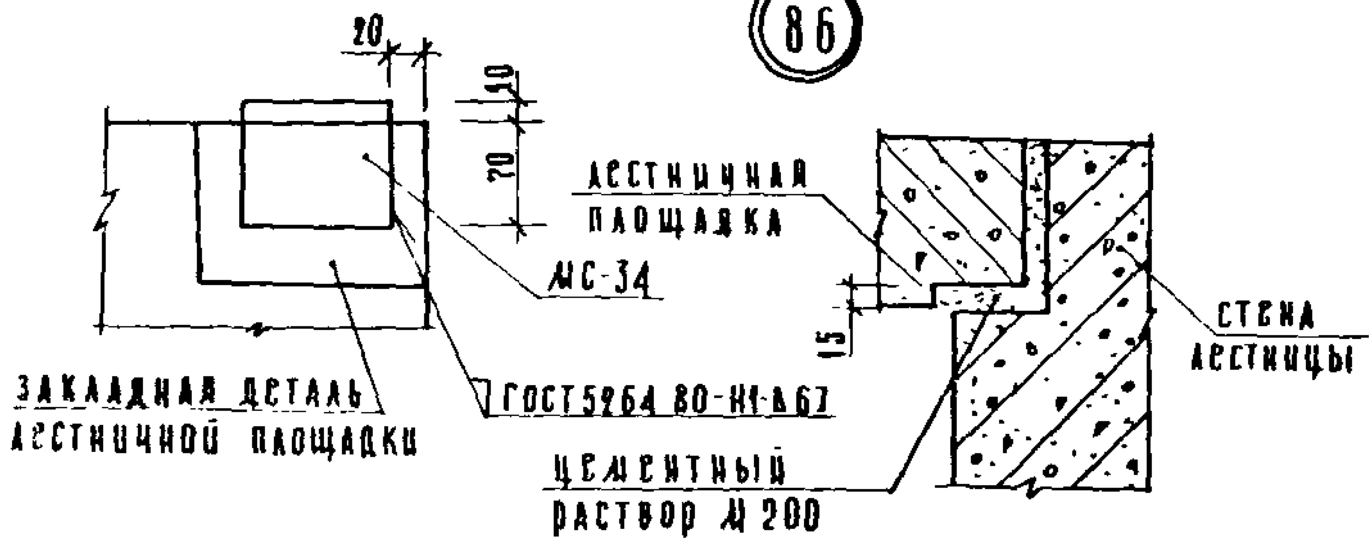
Крепление МС-34 к закладному изделю лестничной площадки
